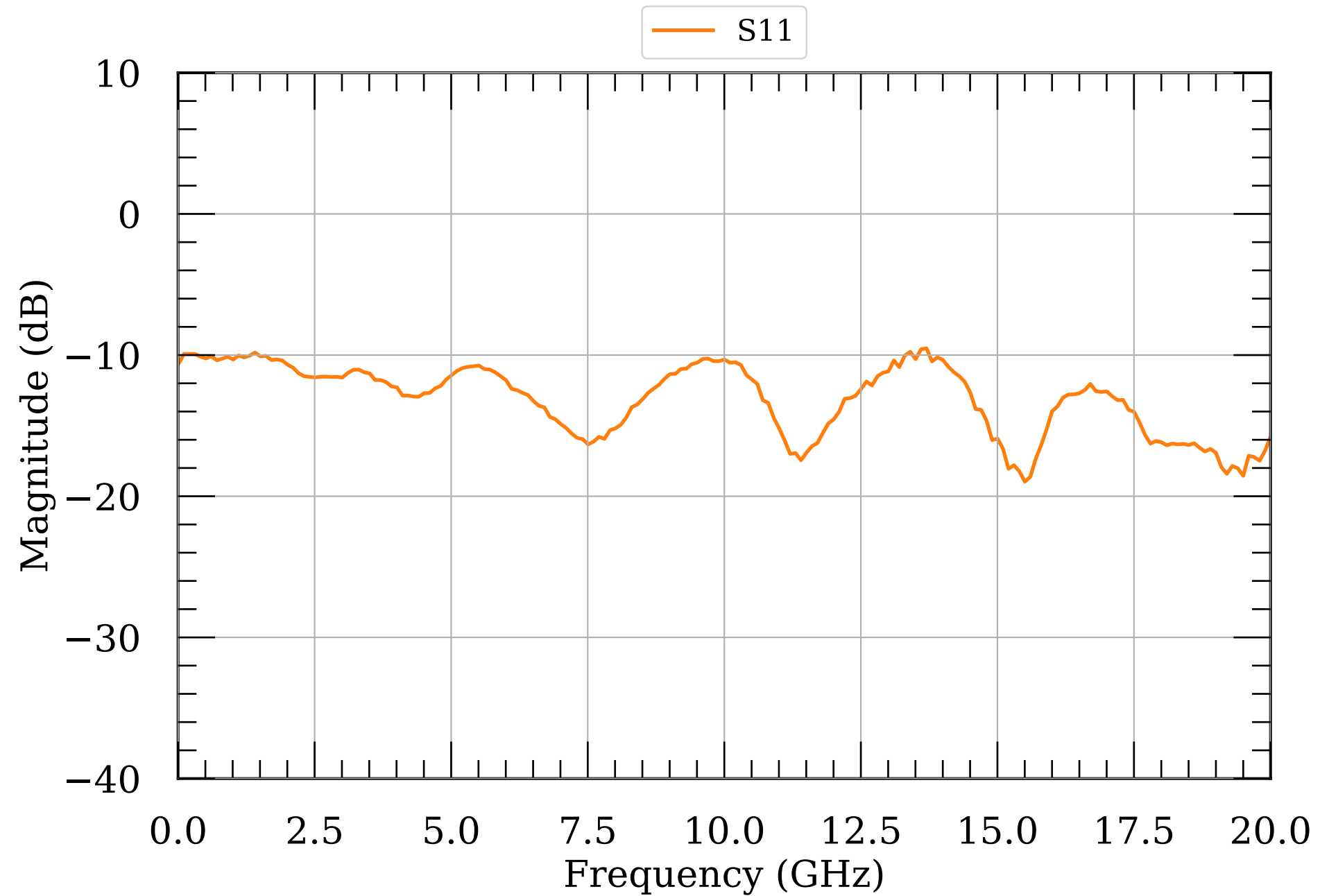
LNA S-params module040v2
